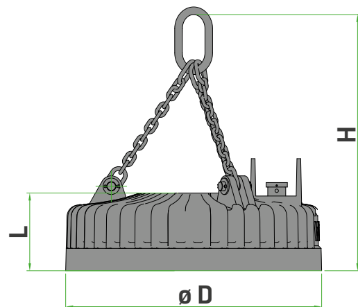
lifting magnet with 3-leg-chain Lasthebemagnet mit 3-Strang-Kette
